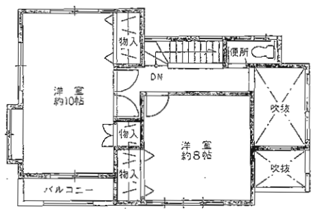
2階平面図
